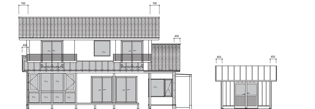
南立面图 1 : 100
