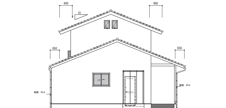
東立面图 1 : 100
