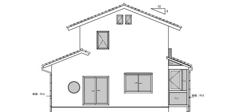
西立面图 1 : 100
