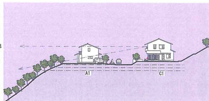
3-3' 立面图
