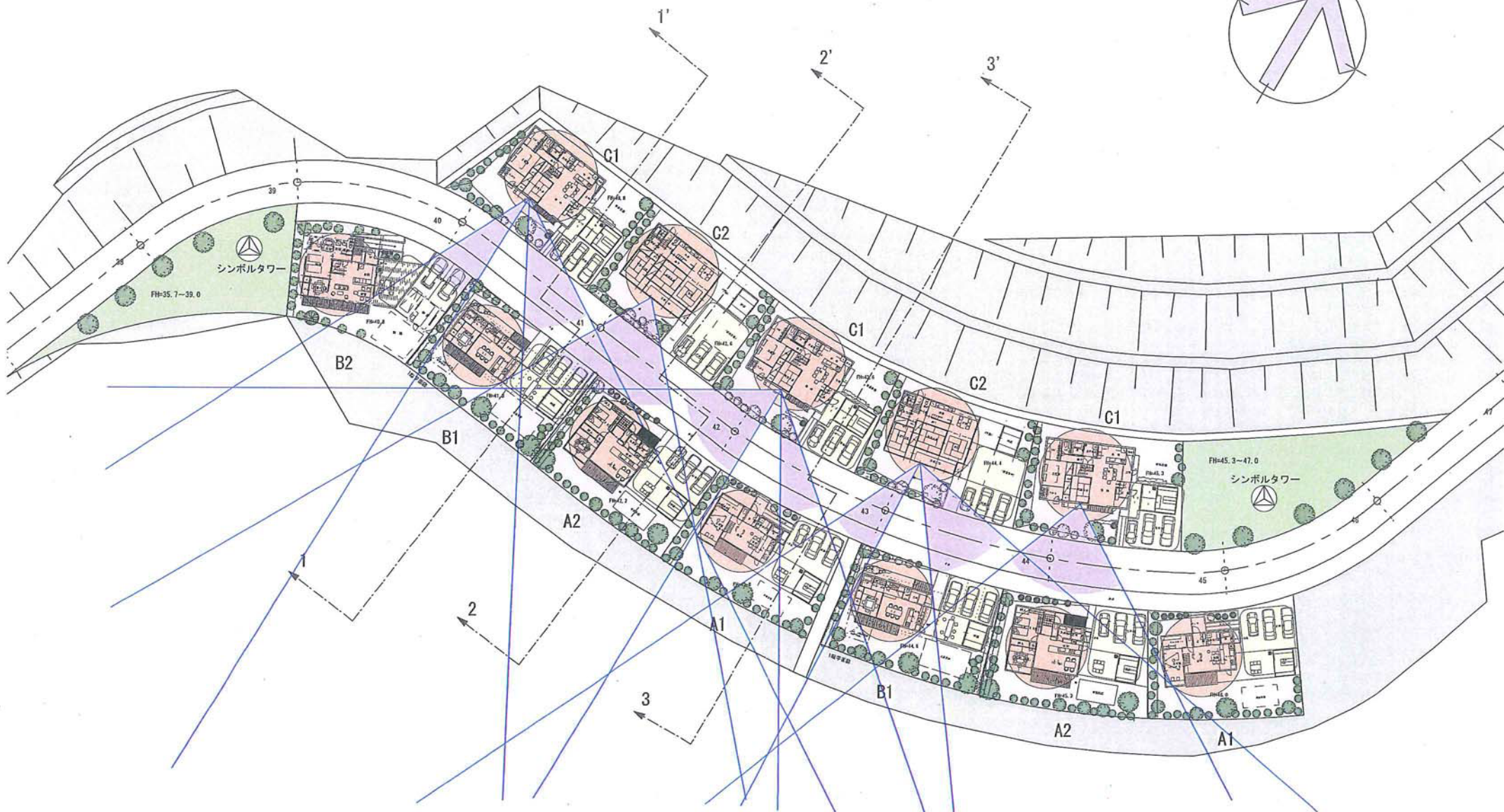
景観検討図 1 : 500
